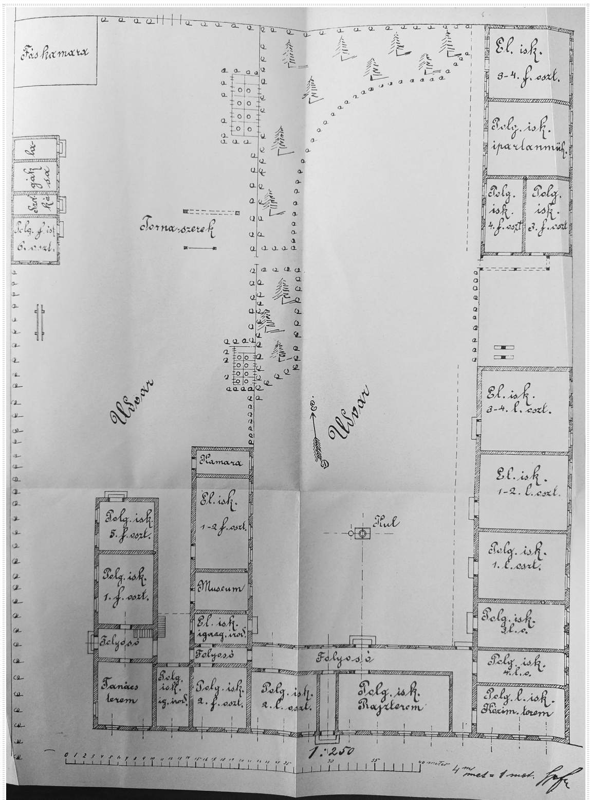
A Nagyszőlősi Magyar Királyi Állami Polgári Fiú- és Leányiskola régi (1908 előtti) épületének alaprajza. (Szerk. Baranyai Gyula: A Nagy-Szőlősi Műasztalossági és... i. m. on.)
