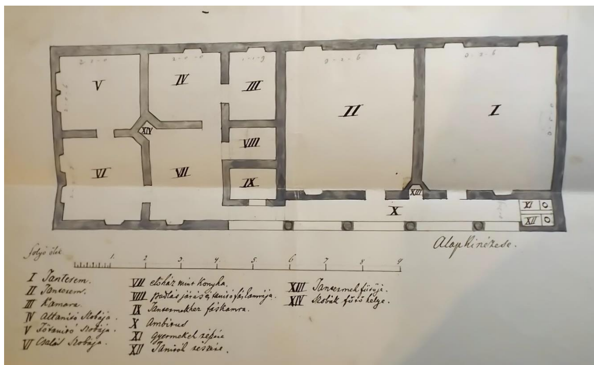
2. kép: Az építendő ecsédi iskola alaprajzának első változata, 1872. (Részlet az Egyházmegyei Hivatal által kiegészített tervrajzból) 780
