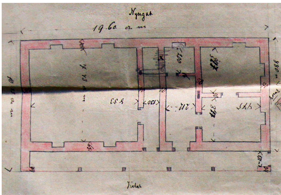
8. kép: A mezőtárkányi harmadik tanterem és tanítói lakás alaprajza, 1888. (Részlet az iskolaépület tervrajzáról) 807
