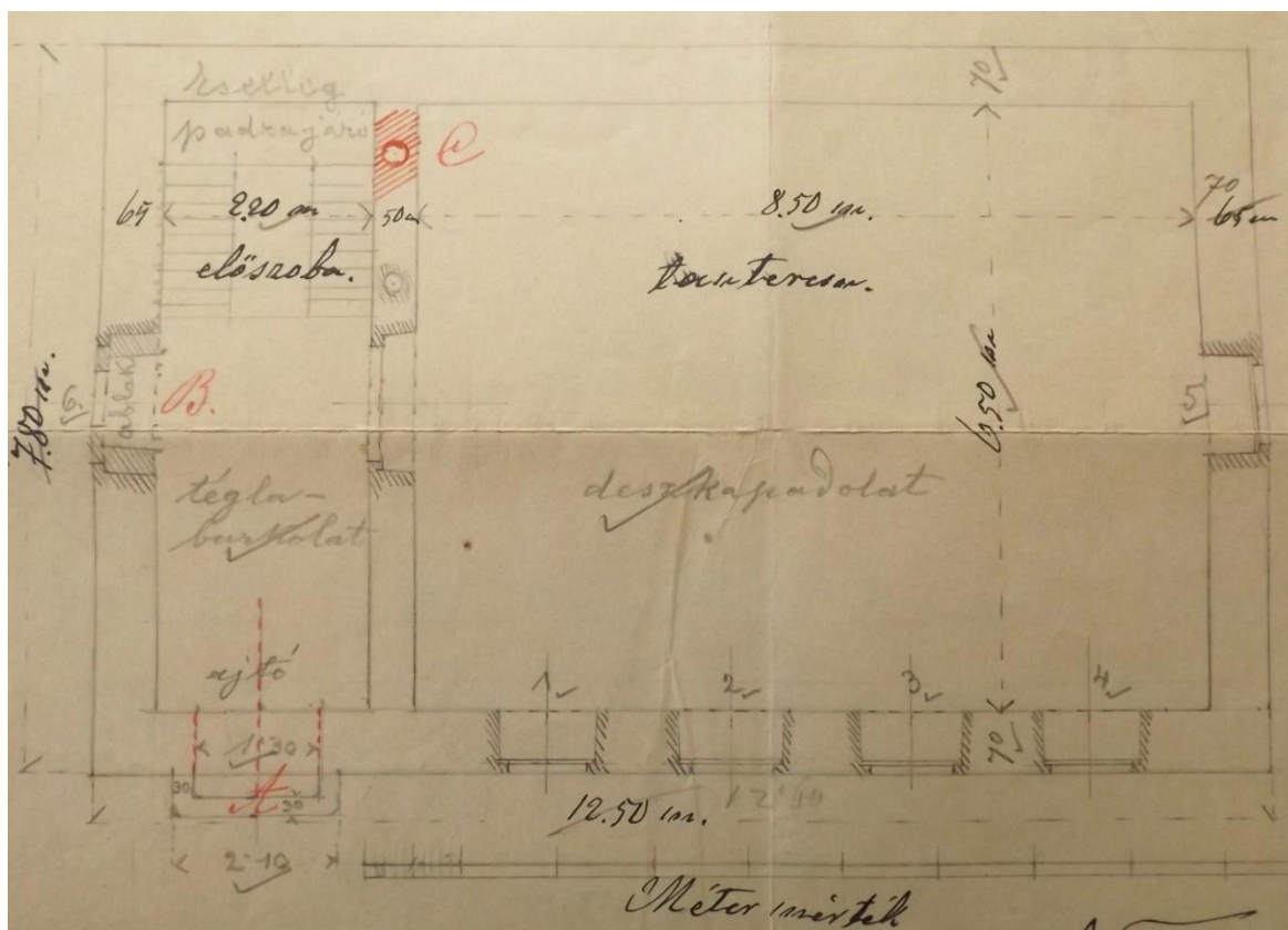
9. kép: A verpeléti iskola negyedik tantermének alaprajza, 1898. (Részlet az iskolaépület tervrajzáról) 832
